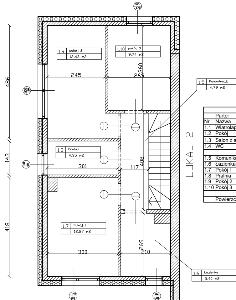
RZUT PIĘTRA
