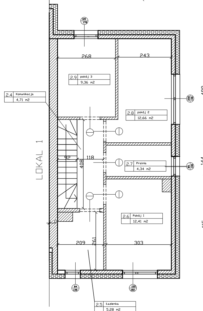
RZUT PIĘTRA
