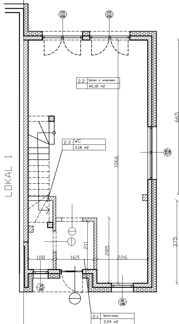
RZUT PARTERU
